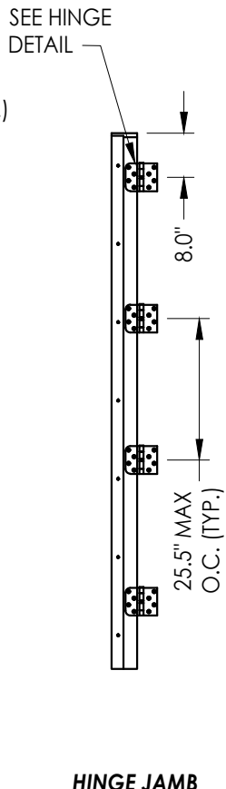
HINGE JAMB
