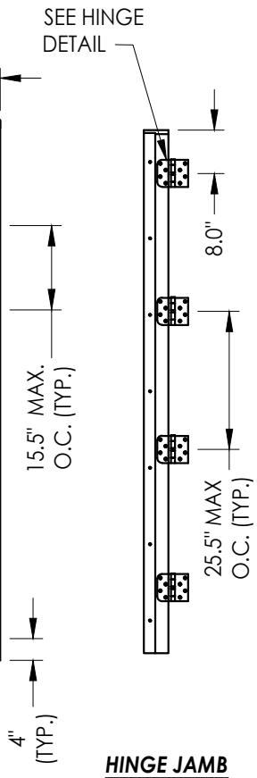
HINGE JAMB
